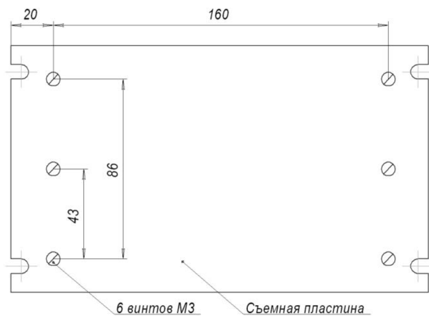
Рисунок Б.2 – Габаритно-установочные размеры БСТ-12Р/380-33-П
